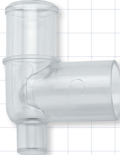
51011 22 mm OD x 22 mm ID x 9 mm ID/12.8 mm OD K-Resin
